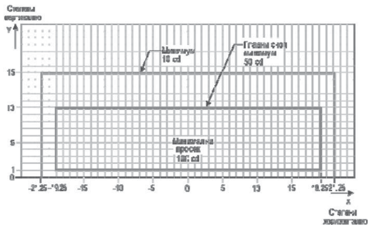
Слика У-18. Изоканделни дијаграм за светла осе рулне стазе (размак 7,5 m) и светла пречке за заустављање на закривљеним деоницама намењена за употребу у условима видљивости дуж полетно-слетне стазе мањој од 350 m
