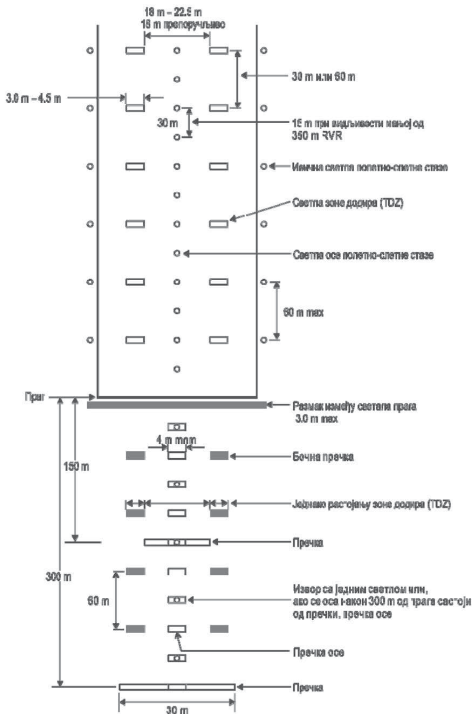
Слика М-3Б. Унутрашњих 300 m прилазних светала и светала полетно-слетне стазе за прецизан прилаз категорија II и III ако постоје задовољавајући нивои употребљивости светала одређени као захтеви одржавања у CS ADR-DSN.S.895
