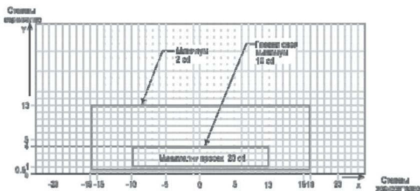
Слика У-19. Изоканделни дијаграм за светла осе рулне стазе (размак 30 m, 60 m) и светла пречке за заустављање на праволинијским деоницама намењена за употребу у условима видљивости дуж полетно-слетне стазе од 350 m или већој
