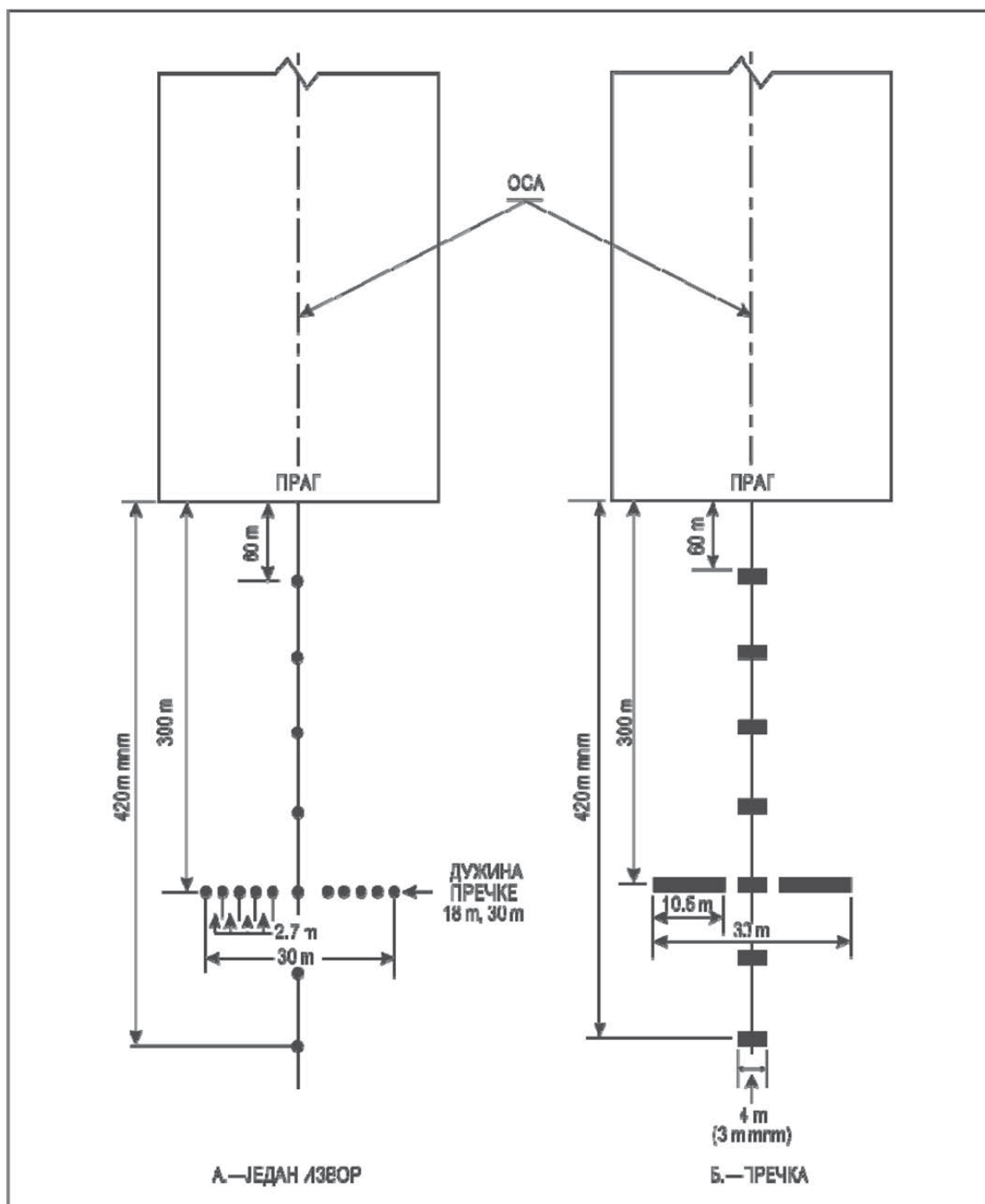
Слика М-1. Једноставни системи прилазних светала
