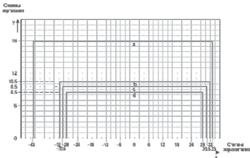
У-23. Изоканделни дијаграм за светла осе рулне стазе (размак 7,5 m) и светла пречке за заустављање високог интензитета на закривљеним деоницама намењена за унапређени систем вођења и контроле кретања по површинама где су потребне веће вредности интензитета светала
