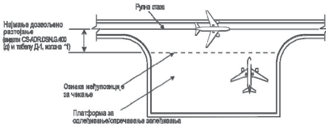
Слика Г-1. Најмање дозвољено растојање на платформи за одлеђивање/спречавање залеђивања ваздухоплова
