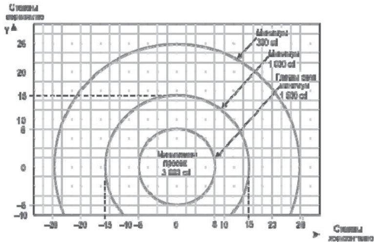
Слика У-28. Изоканделни дијаграм за сваку светилуку заштитних светала полетно-слетне стазе високог интензитета конфигурације А
