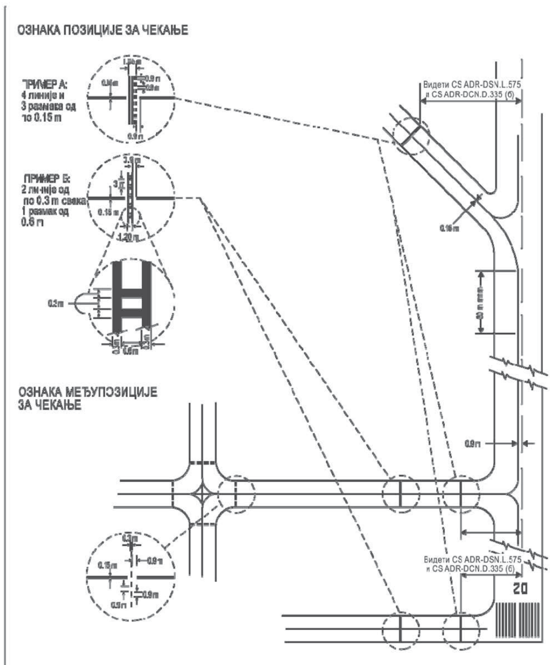
Слика Л-5. Ознаке рулне стазе (приказан са основним ознакама полетно-слетне стазе)
