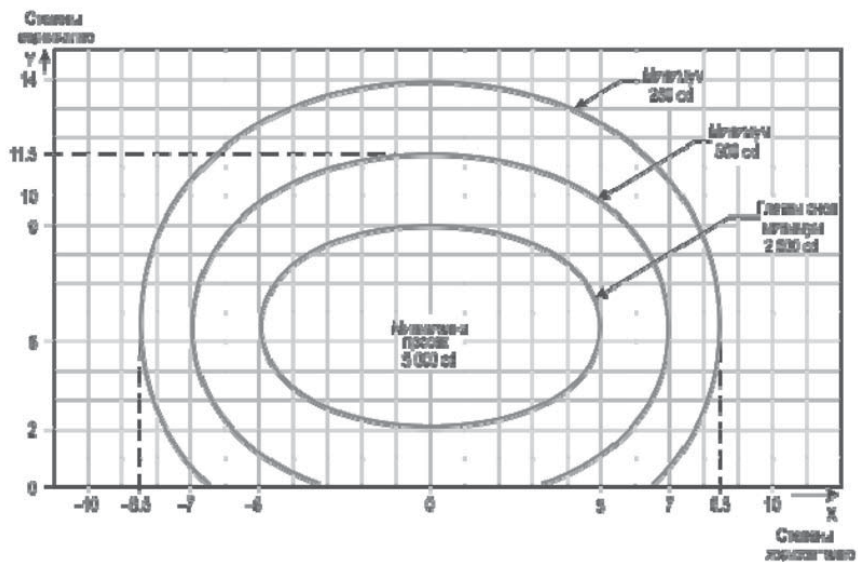
Слика У-9. Изоканделни дијаграм за светло зоне додир (бело светло)
